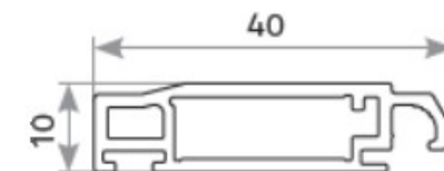
PROFIL A2
