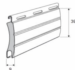
Profil aluminiowy 39 mm
