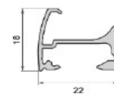
Profil górny/dolny
