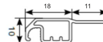
PROFIL MR
