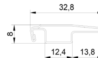
PROFIL UNI
