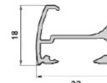
Profil górny/dolny
