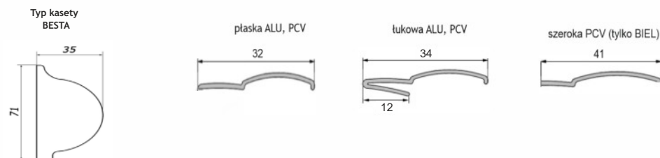
Rodzaje prowadnic
