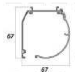
Kaseta B27
