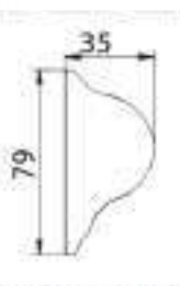
Typ kasety LUX (tylko biel)
