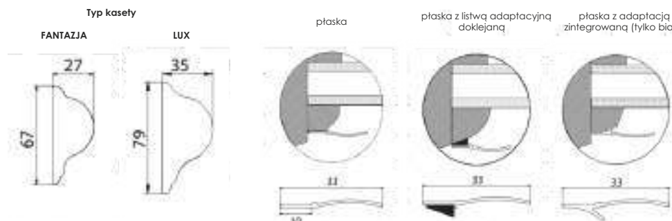
Rodzaje prowadnic
